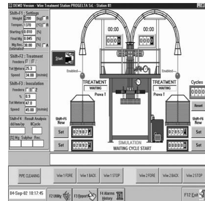
Интерфейс оператора станции модифицирования.
